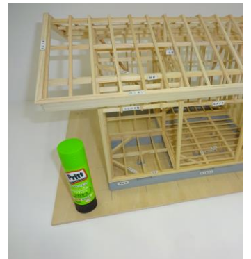
軸組模型
